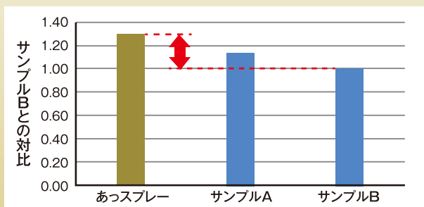
【引張り接着試験】(表層アスコン+基層アスコン)
